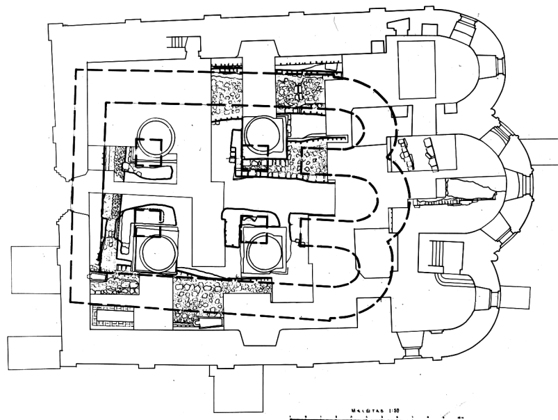
Коломна. Успенский собор. Сводный план шурфов.
