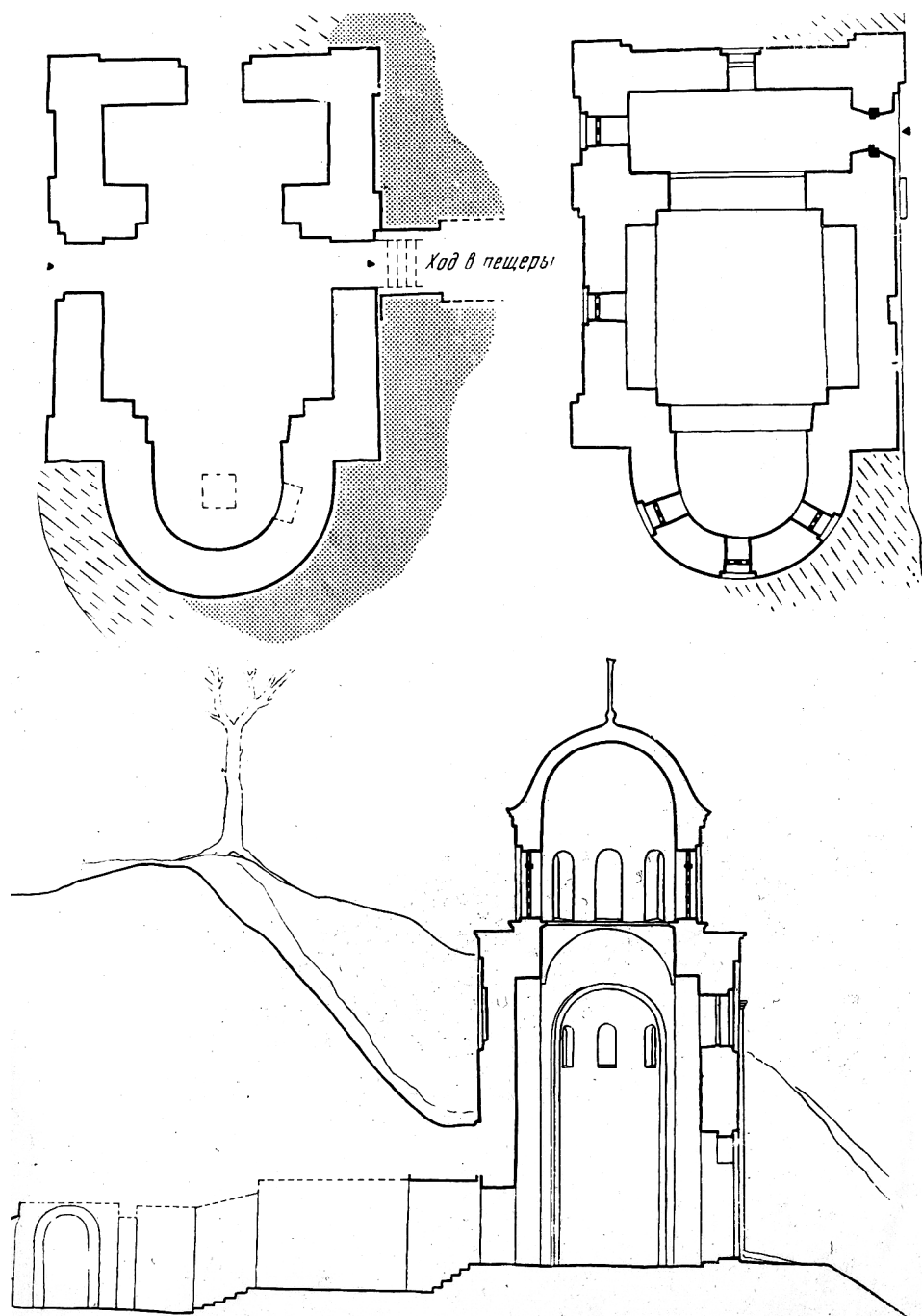
Ильинская церковь в Чернигове. Схема плана по данным 1964 г.
